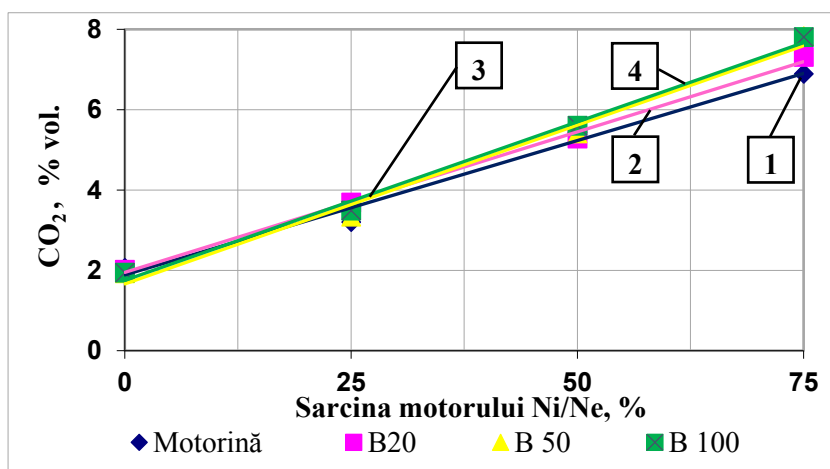
Fig. 6. Frația volumetrică CO 2 în gazele de eșapament funcție de sarcina motorului (1- Motorină; 2 - B20; 3 - B50; 4 - B100; n=2100 min -1 ) (Banari, E., 2022b)
