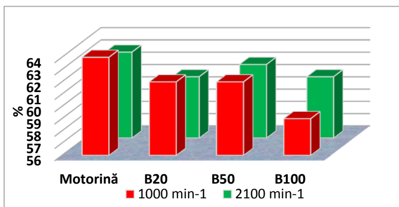
Fig. 8. Valorile emisieii de fum la funcționarea motorului DC4 11,0/12,5 alimentat cu combustibilii cercetați (primul rând n = 1000 \text{ min}^{-1} , al doilea rând n = 2100 \text{ min}^{-1} ) (Banari, E., 2022b)
