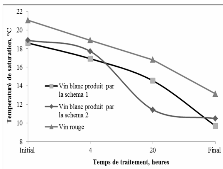
Figure 2. Variation de la température de saturation durant la stabilisation tartrique des vins par la méthode de contact à la température de -5\text{ }^{\circ}\text{C}
