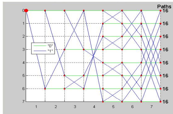
Figura 3. Diagrama trellis
